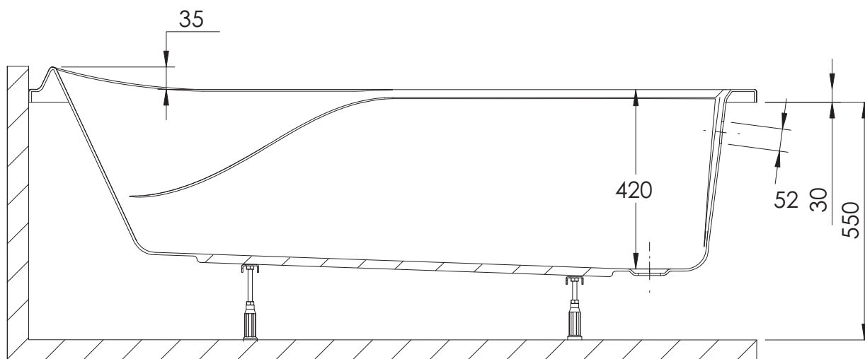
ŘEZ A-A
